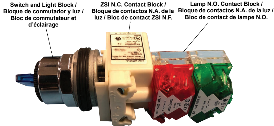
FIG. 2 : MMS Switch Assembly / Montaje del conmutador de MMS / Assemblage du commutateur MMS
