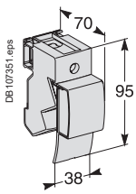
Linergy DX 160 A.
