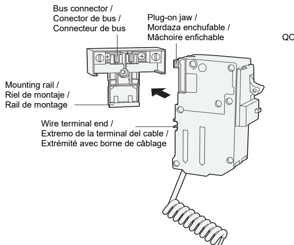
QO Standard Circuit Breaker / Interruptor automático QO estándar / Disjoncteur standard QO
