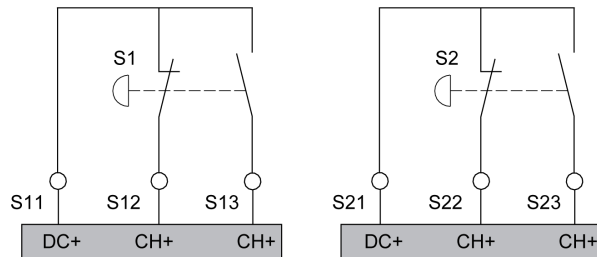
Cableado de las entradas para los dispositivos de control bimanual
