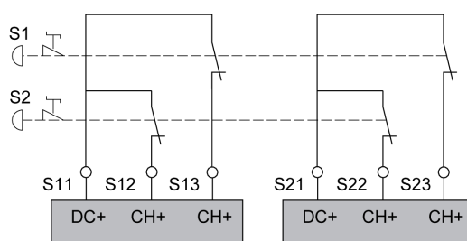
Cableado de las entradas para protecciones
