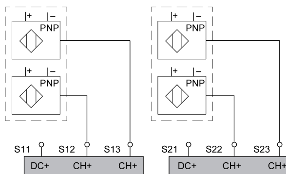
Cableado de las entradas para sensores o dispositivos con dos salidas PNP
