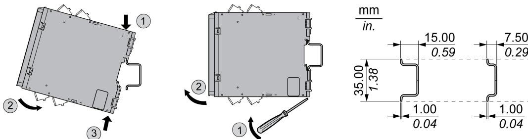
Procedimiento de montaje (ilustración izquierda)
