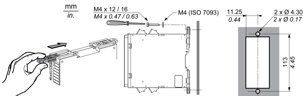
Procedimiento de montaje:
