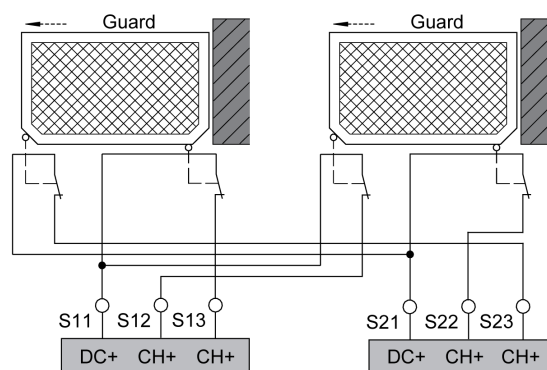
Cableado de las entradas para protecciones
