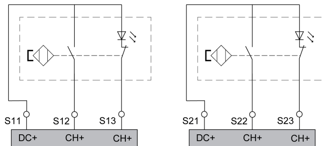
Cableado de las entradas para conmutadores magnéticos codificados
