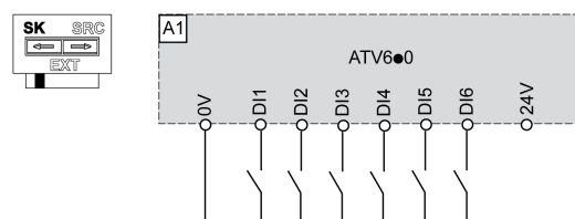
Conmutador en posición SK (sumidero)
