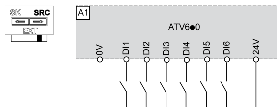
Conmutador en posición SRC (fuente)
