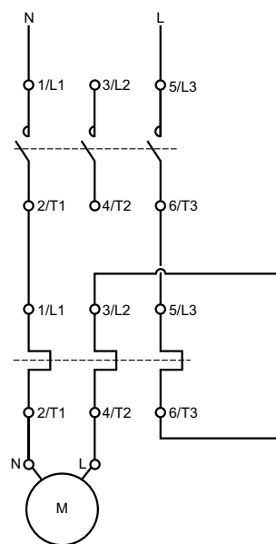
Подключение к автономному реле перегрузки
