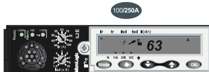
MicroLogic 5 和 6
