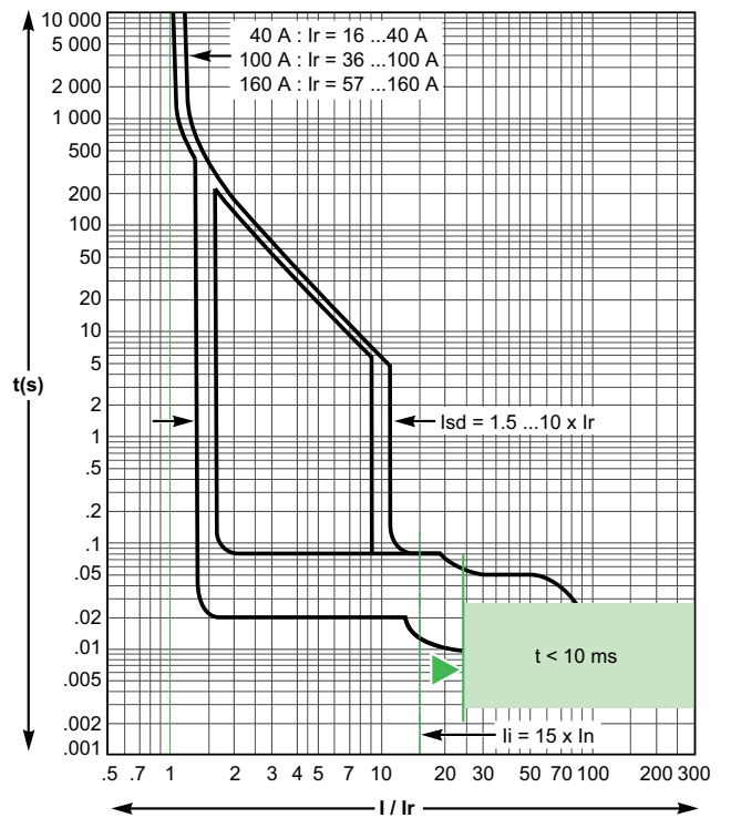
MicroLogic 2.2 和 4.2 - 250 A
