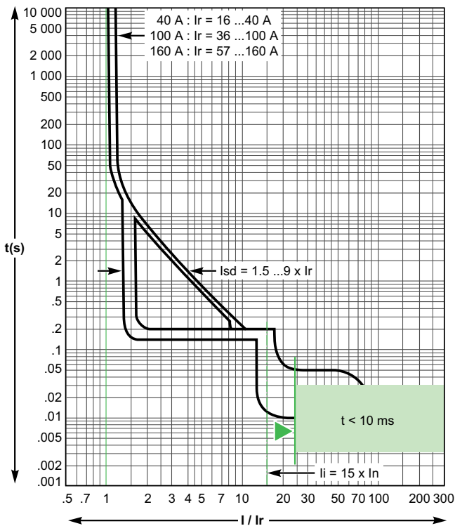
MicroLogic 2.2 和 4.2 - 40-160 A
