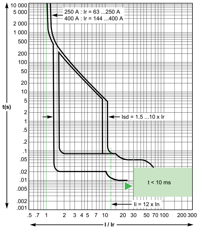
MicroLogic 2.3 和 4.3 - 250-400 A
