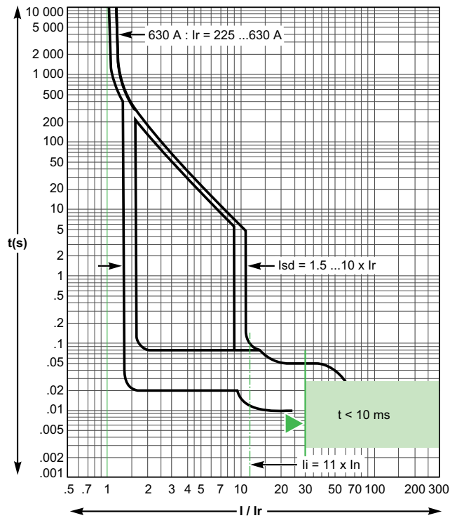
MicroLogic 2.3 和 4.3 - 630 A
