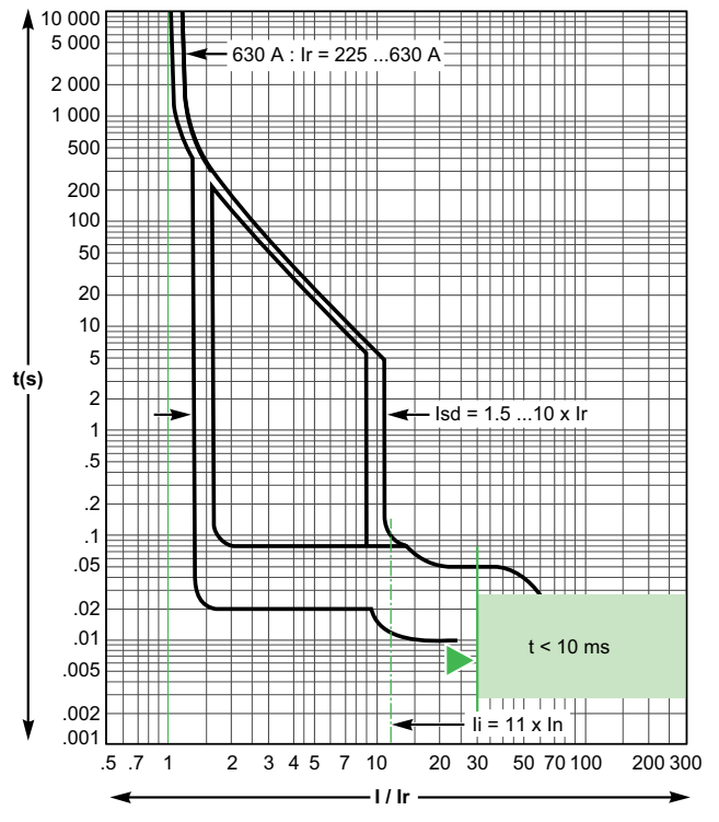
MicroLogic 2.3 和 4.3 - 630 A
