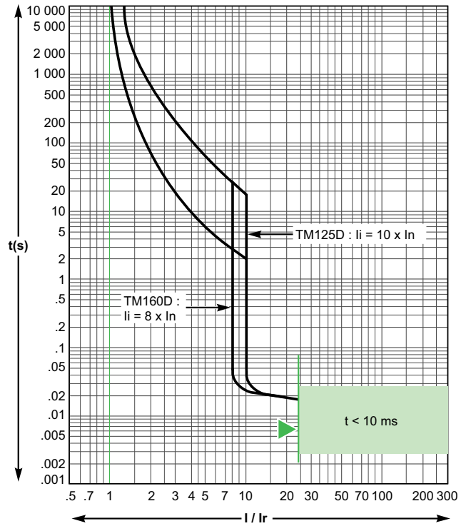
TM125D / TM160D
