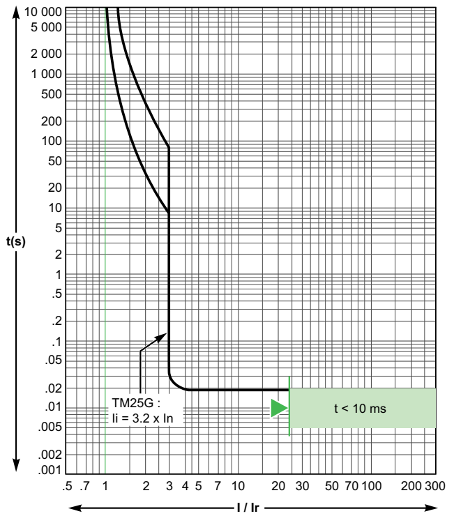
TM25G
