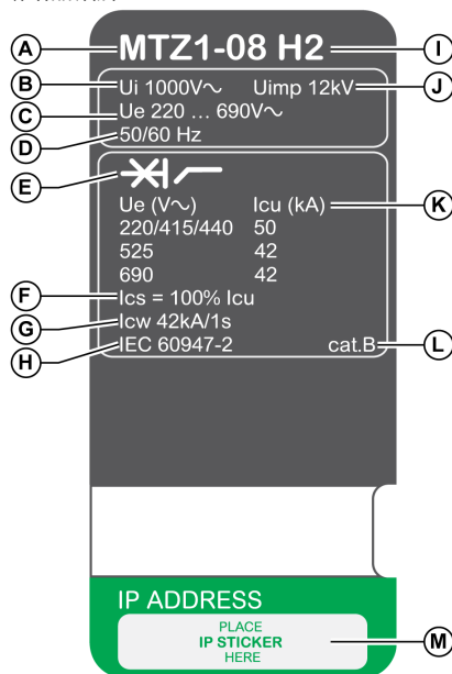
断路器铭牌
