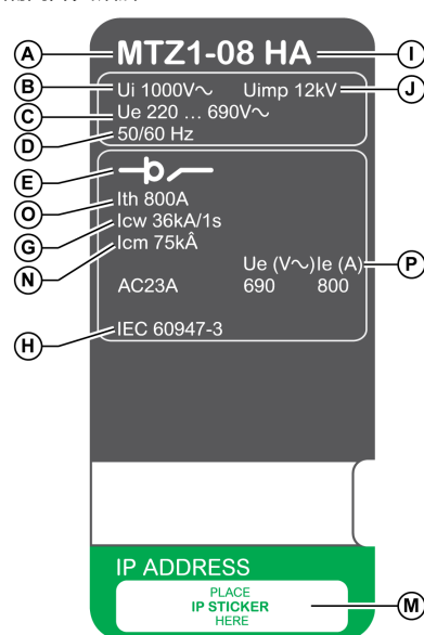
隔离开关铭牌
