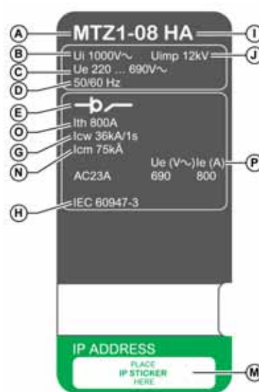
Typenschild Lasttrennschalter
