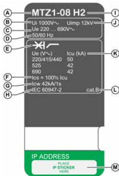
Typenschild Leistungsschalter
