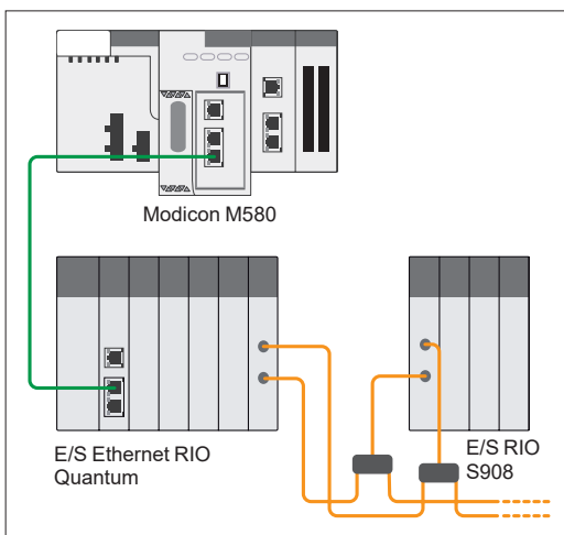
Exemple d'architecture autonome
