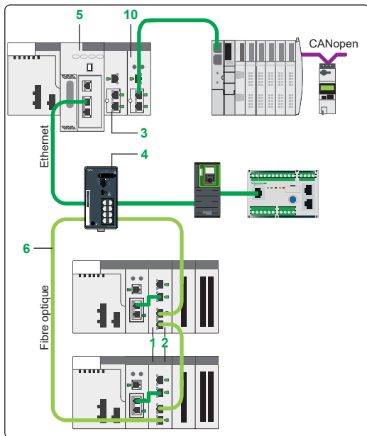
Architecture avec E/S distribuées + architecture avec E/S distantes (avec module switch Ethernet Modicon X80 BMENOS)
