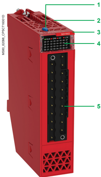
Module d'entrées/sorties TOR de sécurité
