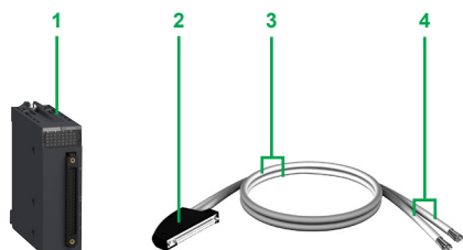
Cordon prééquipé avec connecteur 40 contacts et 2 extrémités fils libres
