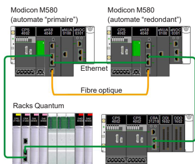
Migration des entrées/sorties Quantum Ethernet
