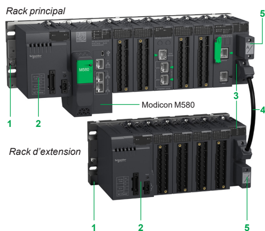
Station avec Modicon M580 sur le rack principal + rack d'extension
