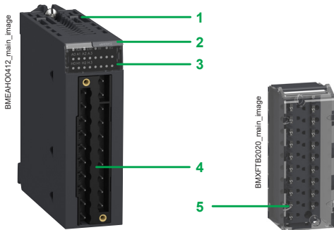
Module à raccordement par bornier débrochable 20 contacts
