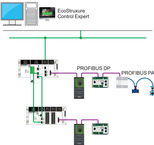
Architecture standard avec utilisation du module PMEPXM0100 dans le rack local et le rack déporté
