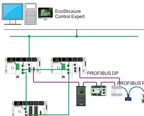
Architecture Modicon M580 à haute disponibilité (HSBY) avec le module PMEPXM0100
