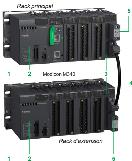
Station avec Modicon M340 sur le rack principal + rack d'extension
