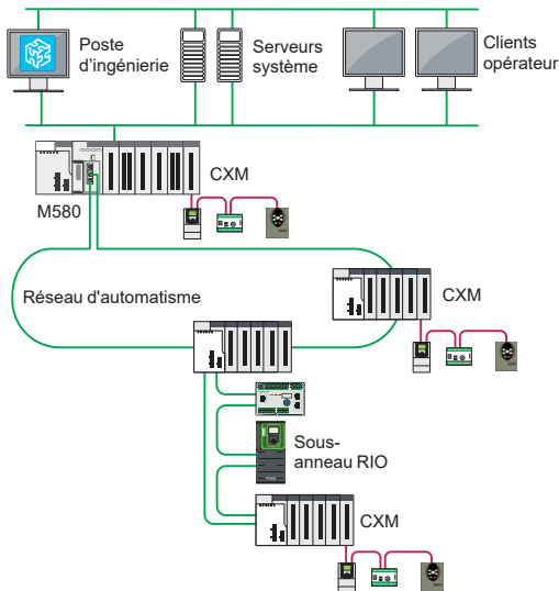
Topologie type pour raccorder des équipements CANopen à une plate-forme Modicon M580 ou une station Modicon X80 à l'aide de BMECXM0100
