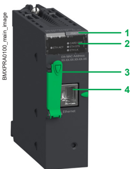
Coupleur Ethernet pour rack E/S distribué Modicon X80
