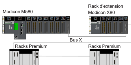
Exemple d'extension bus X Premium
