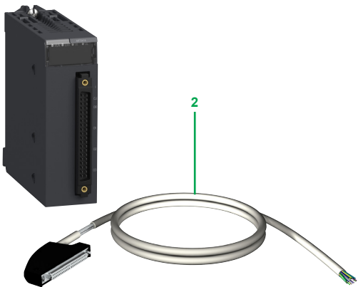
Cordon BMXFCW●01S (avec connecteur 40 contacts et extrémité fils libres)
