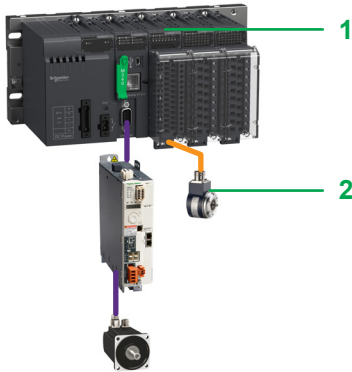
Plate-forme Modicon X80 avec processeur Modicon M340
