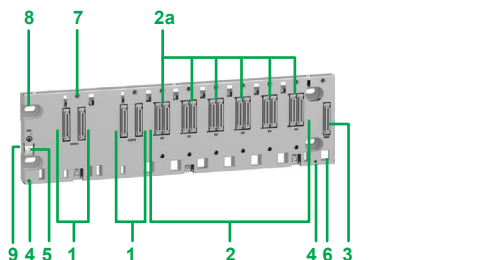
Fond de panier BMEXP0602
