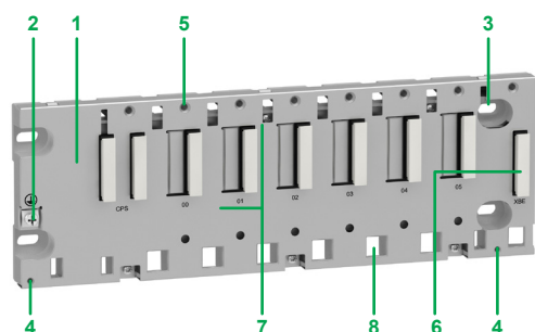
Fond de panier à 6 emplacements BMXXBP0600
