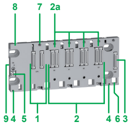
Fond de panier BMEXBP0400
