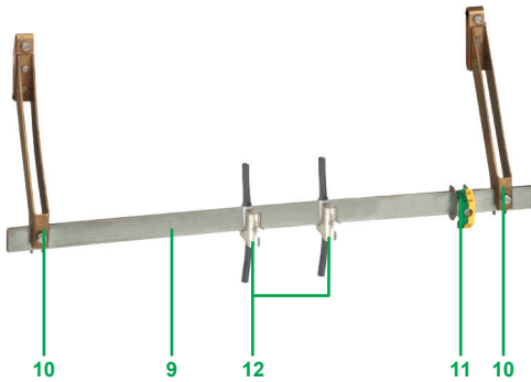
Kit de reprise de blindage des câbles BMXXSP●●00
