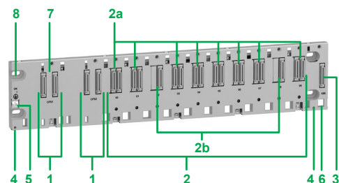
Fond de panier BMEXP1002
