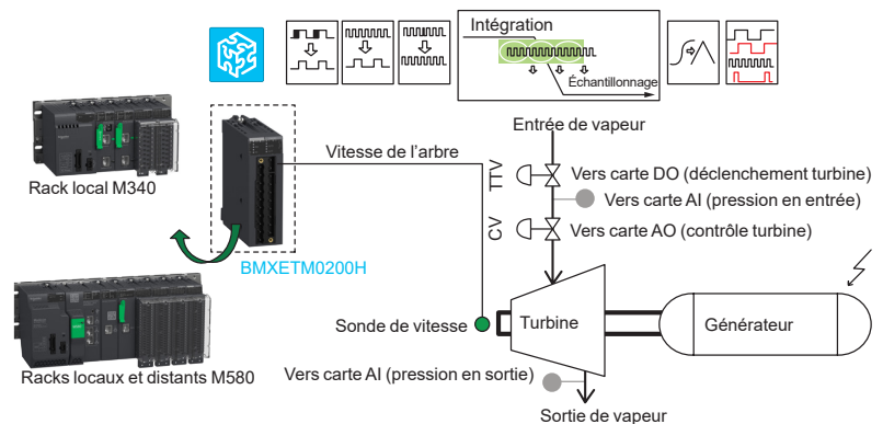
Architecture d'un système de contrôle de régulateur TMC
