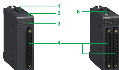
Modules 32 voies et 64 voies à raccordement par 1 ou 2 connecteurs 40 contacts
