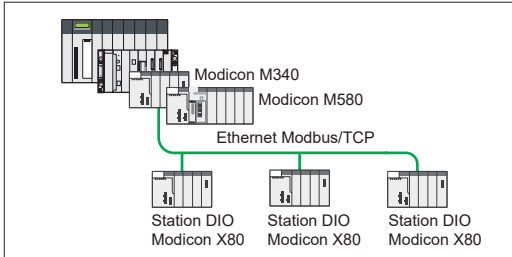
Stations DIO Modicon X80 dans un réseau Ethernet Modbus/TCP
