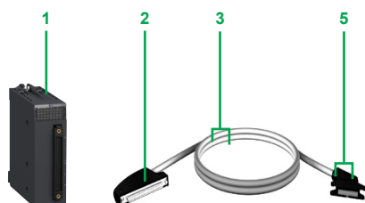
Cordon prééquipé avec connecteur 40 contacts et connecteur HE10 pour système Modicon ABE7 Telefast
