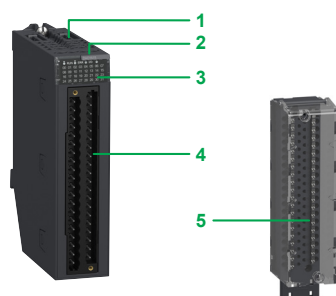
Module à raccordement par bornier débrochable 20 contacts
