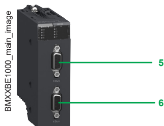
Module d'extension rack BMXXBE1000
