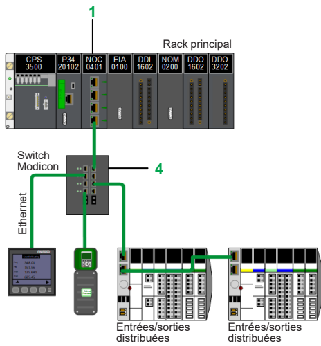
Architecture d'entrées/sorties distribuées avec BMXNOE0110
