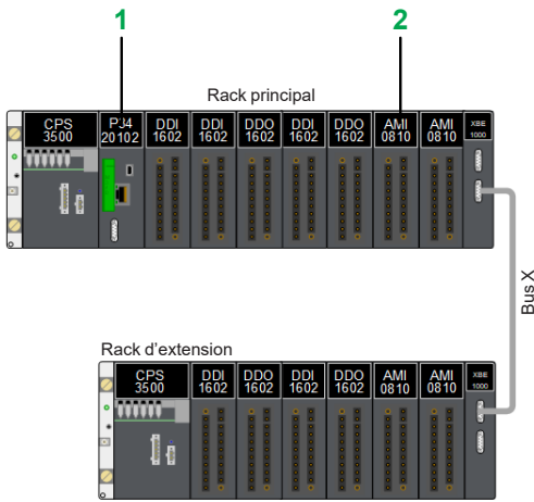
Architecture d'entrées/sorties locales
