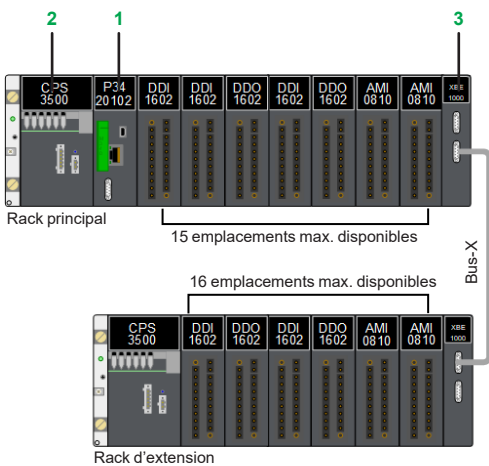
Architecture d'entrées/sorties locales
