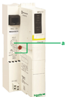
Module réseau NIM des entrées/sorties Modicon STB
