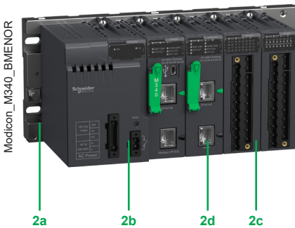
Modules Modicon X80
