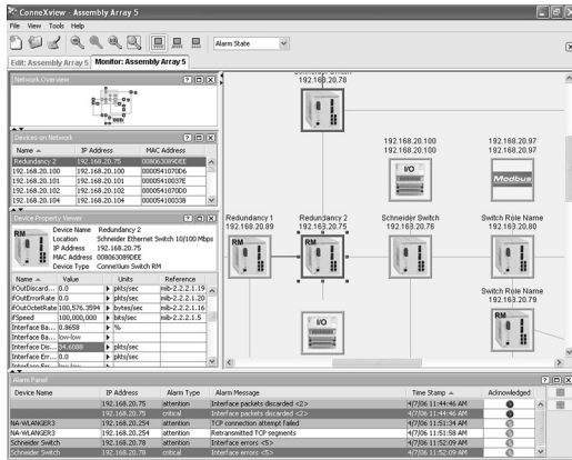
Détection automatique des équipements IP via le logiciel ConneXview de diagnostic des réseaux industriels Ethernet
