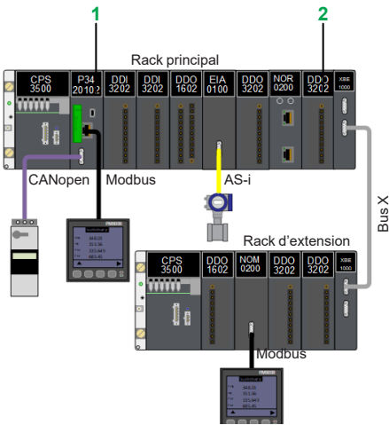
Architecture de bus de terrain intégré
