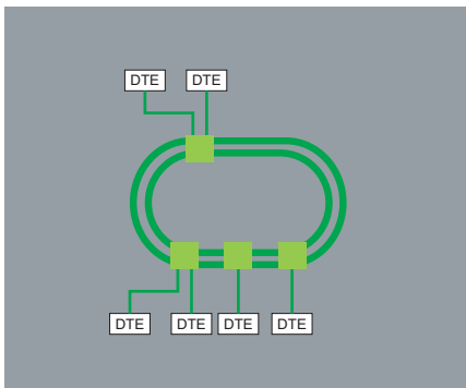
Topologie en anneau double
