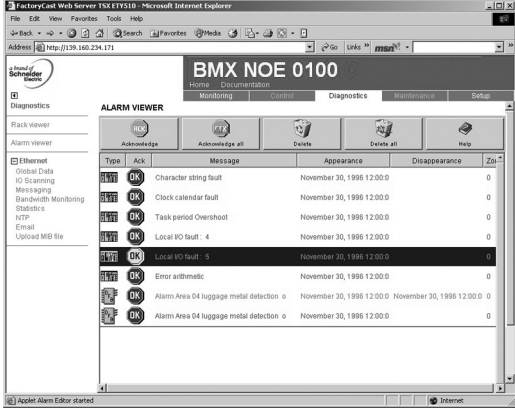
Visualisation d'alarmes à partir du buffer de diagnostic
