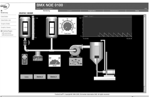
Interface graphique de conduite temps réel
