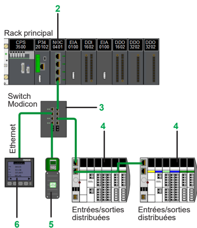
Architecture d'entrées/sorties distribuées : équipements distribués sur Ethernet avec module BMXNOC0401 et switch Modicon
