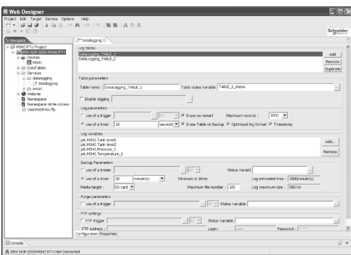
Configuration de la fonction "Data Logging" pour le module BMXNOR0200H
