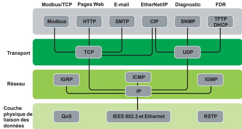
Services de communication Ethernet du module BMXNOE0100/0110
