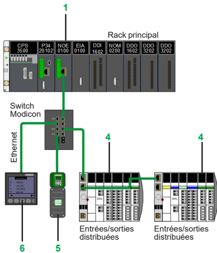
Architecture d'entrées/sorties distribuées : équipements distribués sur Ethernet avec module BMXNOE0100 et switch Modicon
