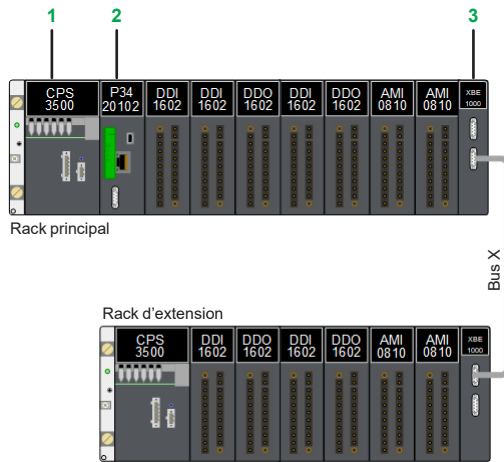
Architecture d'entrées/sorties locales : équipements sur entrées/sorties locales
