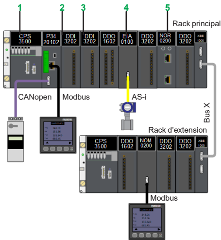
Architecture de bus de terrain intégré : équipements distribués sur bus de terrain
