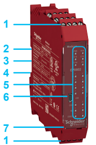
Composants de sécurité
