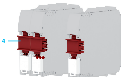
Connecteurs d'extension en fond de panier
