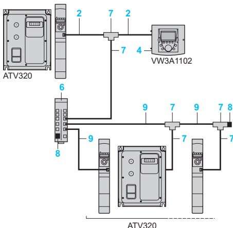
Exemple d'un raccordement multipoint
