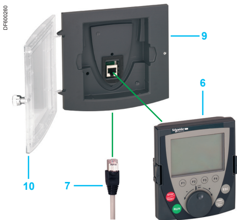
Déport du terminal graphique sur porte d'enveloppe : 6 + 7 + 9 si IP 54, 6 + 7 + 9 + 10 si IP 65
