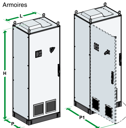
VLVAF6P Armoires
