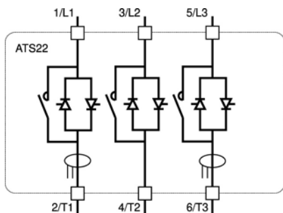
Gamma ATS22●●●Q
