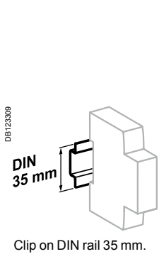
Clip on DIN rail 35 mm.
