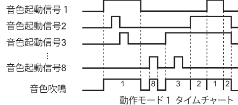
動作モード1 タイムチャート
