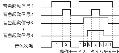
動作モード2 タイムチャート
