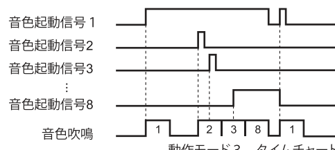
動作モード3 タイムチャート
