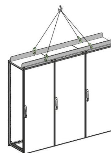
Elevação
