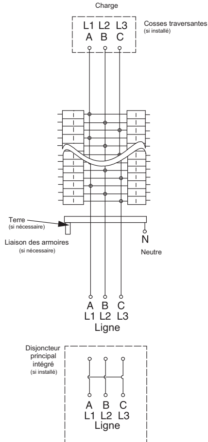
Figure 8 - Schéma de cosses principales ou disjoncteur principal (avec ou sans cosses traversantes) NF 400-800 A pour panneaux de distribution NQ ou centre de charge QONQ
