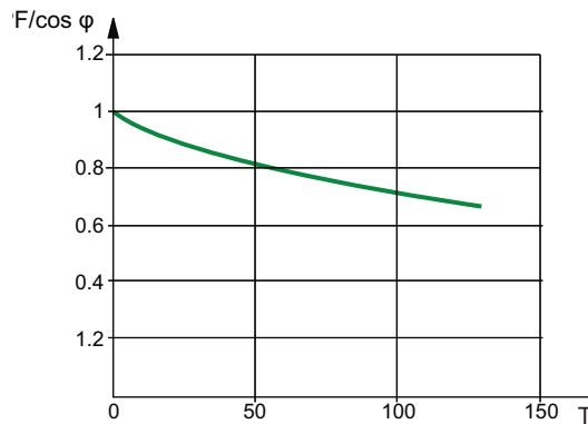
Figura 19 – PF/Cos \varphi como una función de THD(I)
