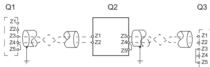
Figura 14 – Alambrado de ZSI
