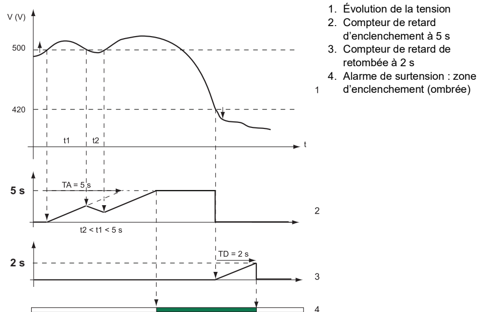
Figure 25 – Retard sur une alarme de surtension
