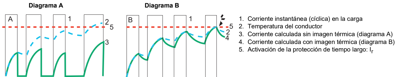
Figura 6 – Diagramas de elevación de la temperatura del conductor
