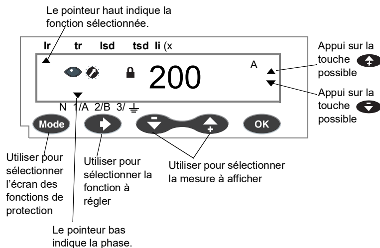
Figure 3 – Écran des fonctions de protection
