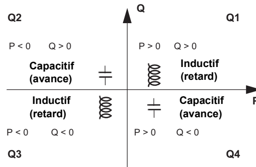
Figure 17 – Quadrants de fonctionnement (Q1, Q2, Q3 et Q4)
