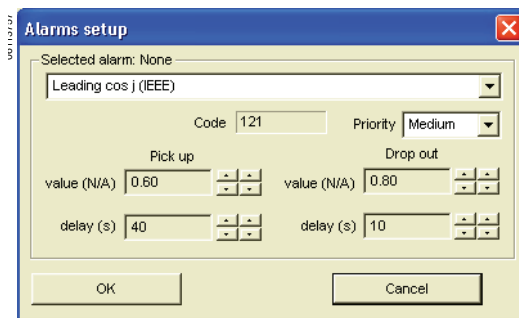
121 supervisando el cos φ capacitivo
