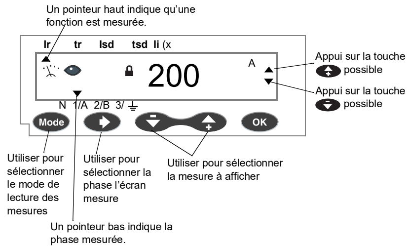
Figure 1 – Écran de lecture
