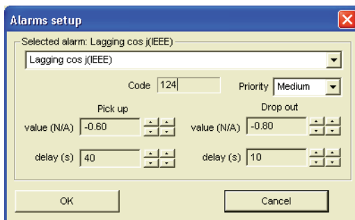
124 supervisando el cos φ inductivo
