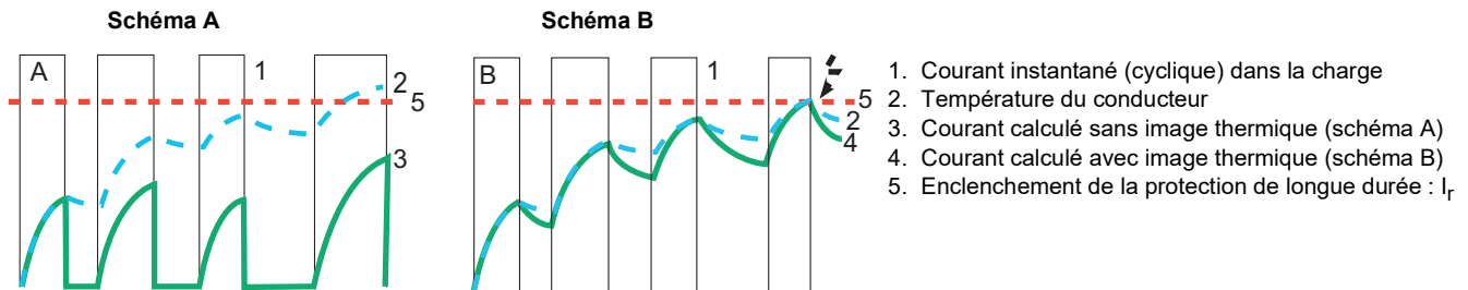
Figure 6 – Schémas de l'échauffement d'un conducteur
