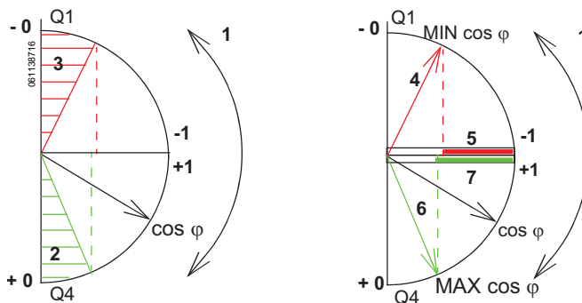
Figura 21 – Cos φ Indicador
