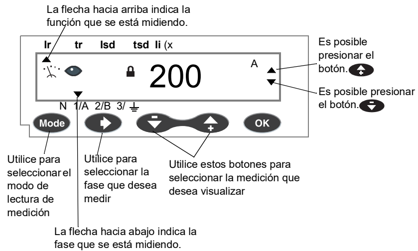
Figura 1 – Pantalla de lectura
