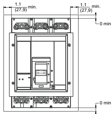
FIG. 1 : Minimum Clearance to Metal / Requisitos de espacio libre mínimo con piezas de metal / Exigence d'espace minimum avec du métal
