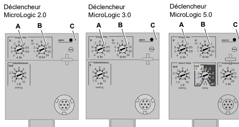
Figure 5 – Commutateurs de protection de longue durée
