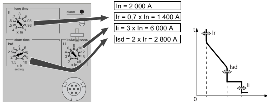
Figura 16 – Ajuste del retardo
