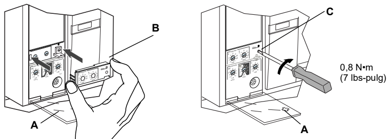
Figura 22: Instalación del calibrador ajustable
