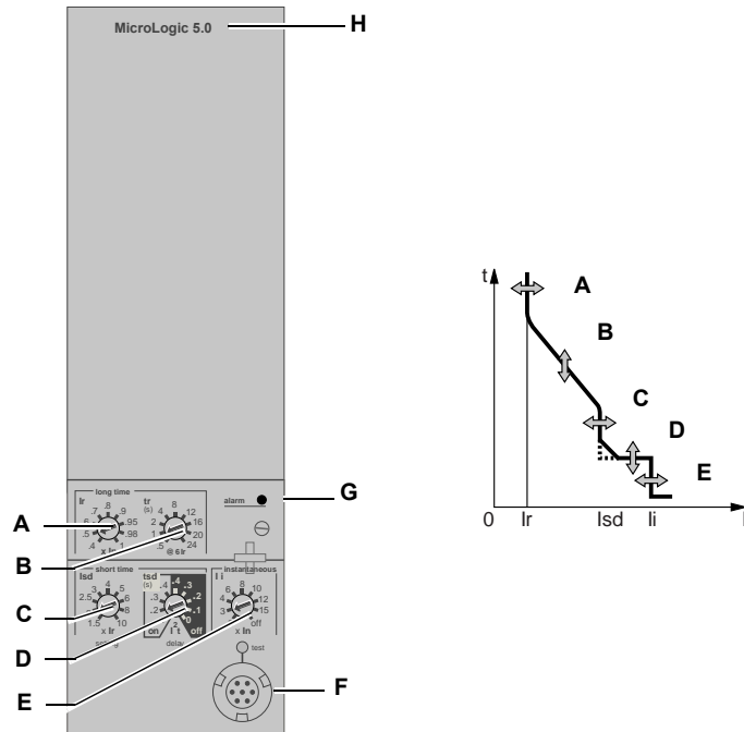
Figura 4: Ajustes y curva de disparo para la unidad de disparo 5.0
