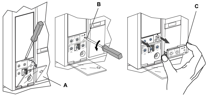
Figura 18: Desmontaje del calibrador ajustable
