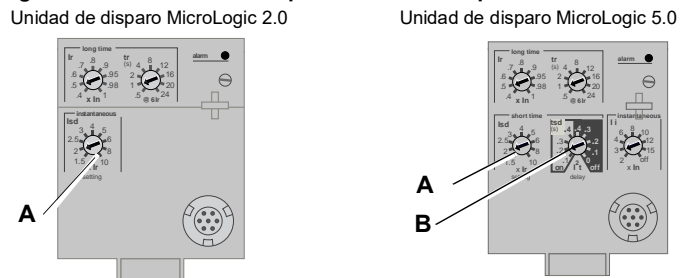
Figura 6: Selectores de protección de tiempo corto
