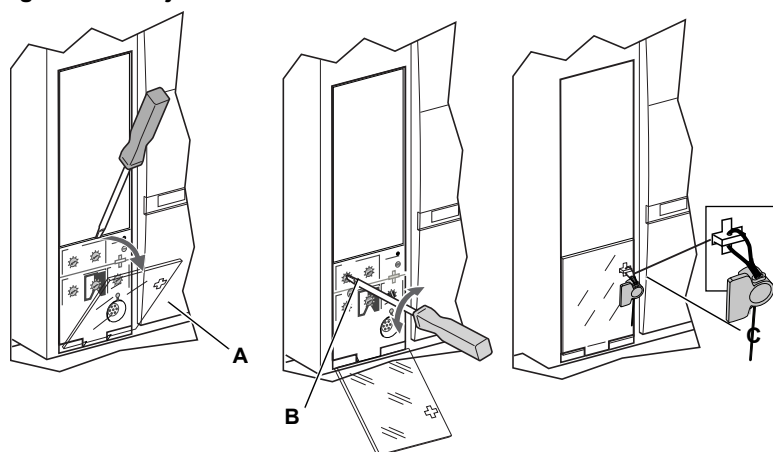
Figura 9 – Ajuste los valores de los selectores
