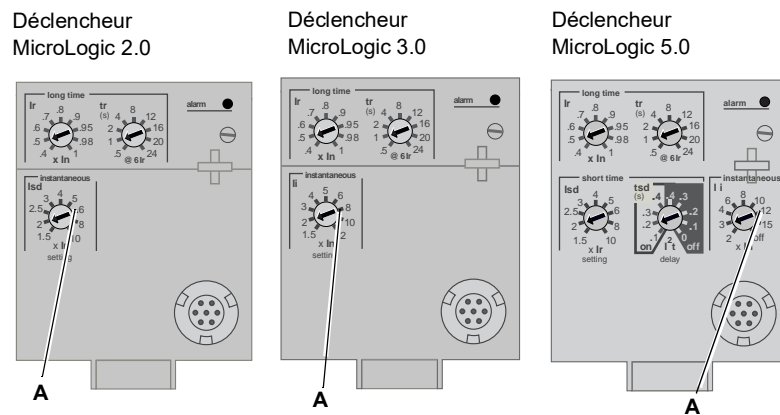
Figure 7 – Commutateurs de protection instantanée
