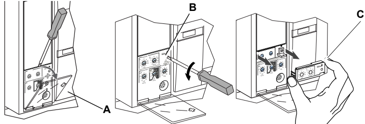
Figura 23: Desmontaje del calibrador ajustable
