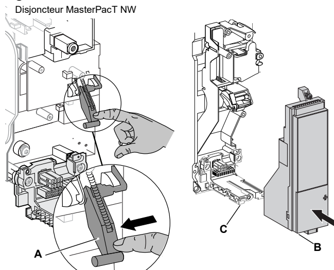
Figure 20 – Installation du déclencheur
