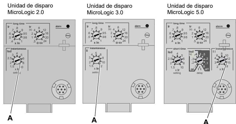
Figura 7: Selectores de protección instantánea
