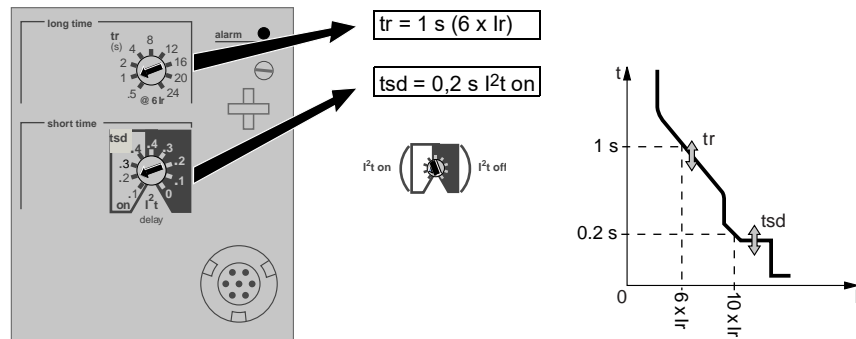
Figura 16 – Ajuste del retardo
