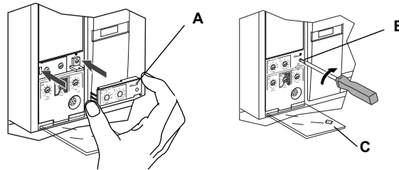
Figure 24 : Installer la nouvelle fiche de valeur nominale réglable
