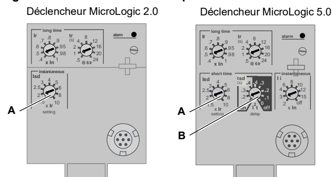
Figure 6 – Commutateurs de protection de courte durée
