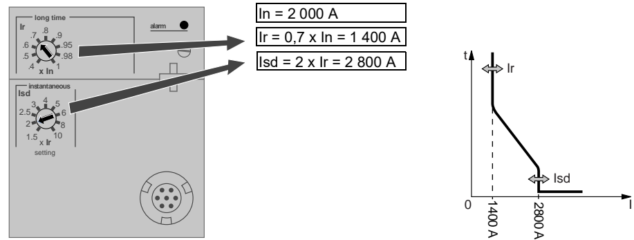
Figura 11 – Ajuste de los niveles de activación
