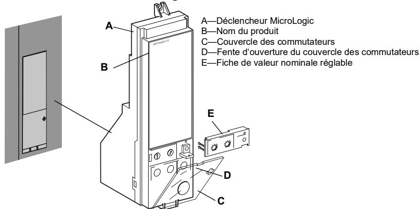
Figure 1 – Déclencheur MicroLogic
