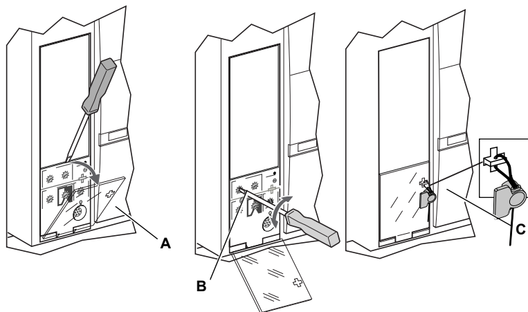
Figure 9 : Affinement des réglages des commutateurs
