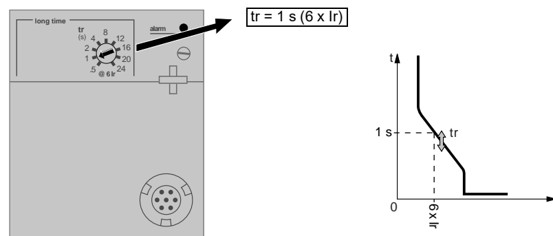
Figura 12 – Ajuste del retardo
