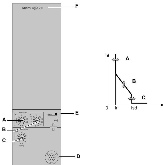
Figure 2 – Réglages et courbe de déclenchement pour le déclencheur 2.0
