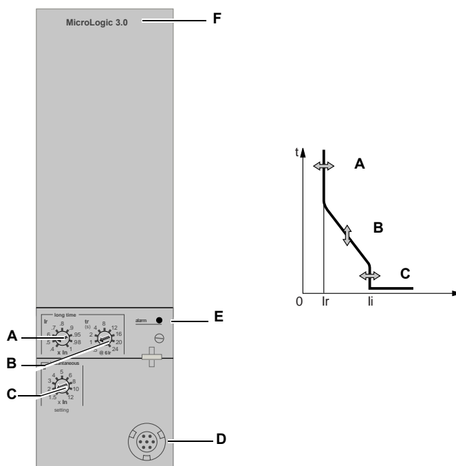
Figure 3 – Réglages et courbe de déclenchement pour le déclencheur 3.0
