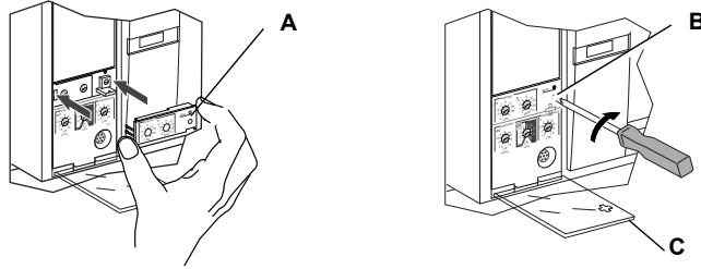
Figura 24: Instalación del nuevo calibrador ajustable
