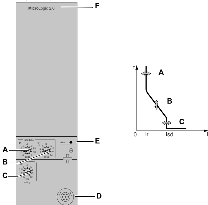
Figura 2: Ajustes y curva de disparo para la unidad de disparo 2.0
