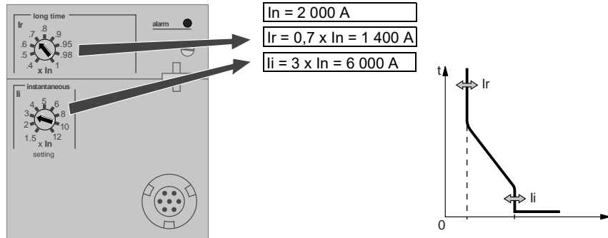
Figura 13 – Ajuste de los niveles de activación
