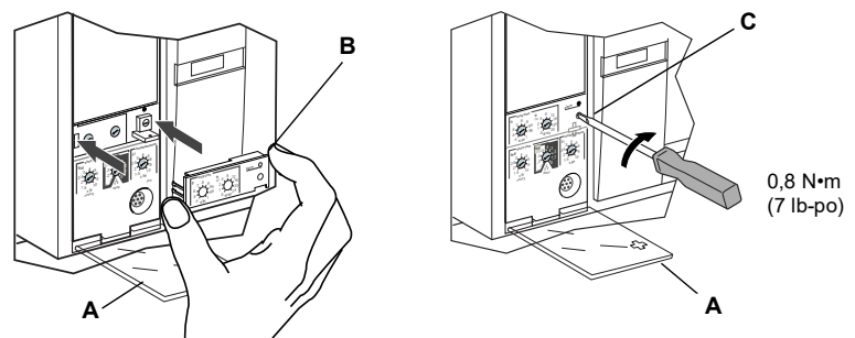
Figure 22 – Installation de la fiche de valeur nominale réglable
