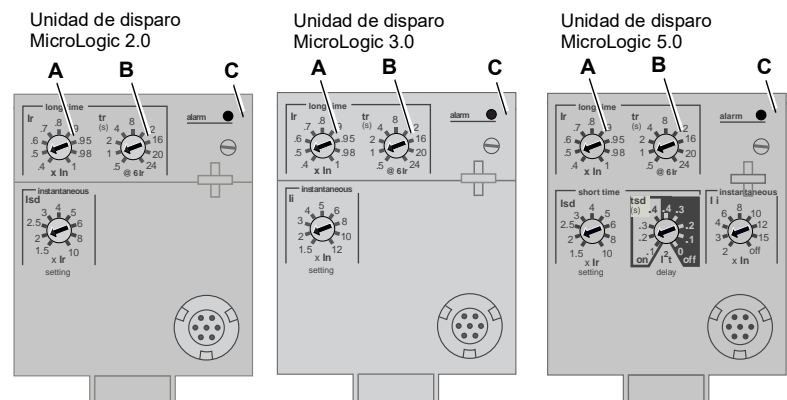
Figura 5: Selectores de protección de tiempo largo
