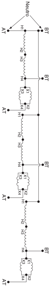
Diagrama de alambrado 9
