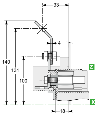
NSX100 à 250
