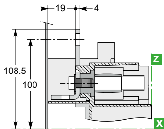
NSX100 à 250
