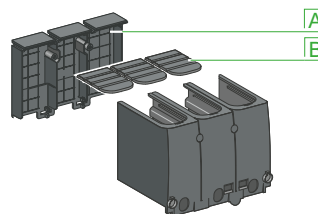
A Repères de prédécoupe
