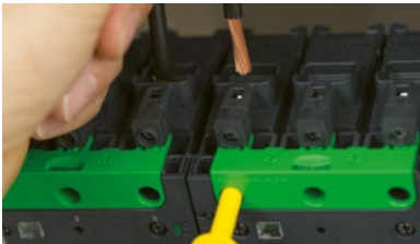
Amélioration de l'efficacité de câblage Connexions fiables avec technologies EverLink™ brevetées et éprouvées.
