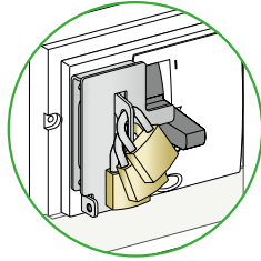
Verrouillage à maneton à l'aide de cadenas et d'un accessoire :
