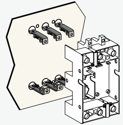
Raccordement prise arrière avec fixation sur panneau arrière.
