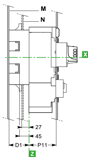
Commande par maneton
