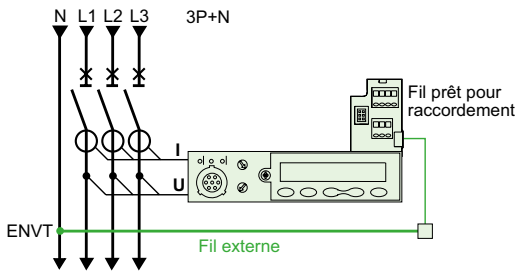
Prise de tension neutre externe (ENVT).
