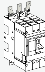
Raccordement prise avant avec épanouisseur.
