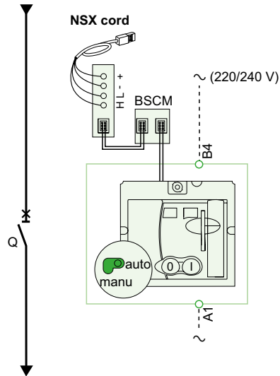
Représentation schématique du réarmement communicant (MT).
