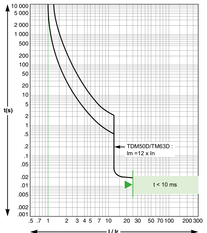
TM50D / TM63D
