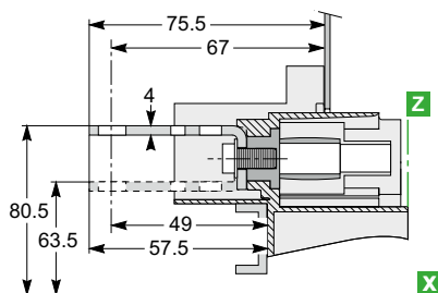
NSX100 à 250
