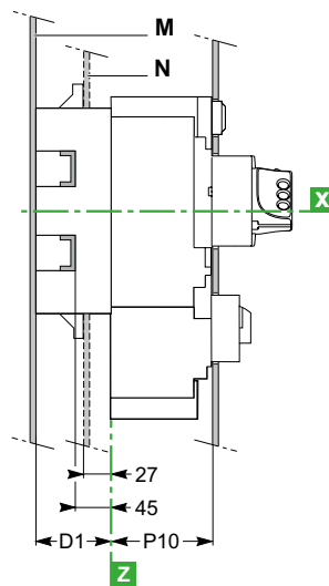
Poignée rotative
