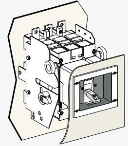
Cadre de porte standard avec collier pour retrait, pour maneton.
