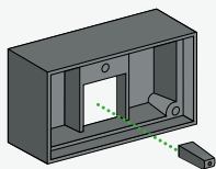
Collier de protection pour une poignée et une extension de poignée afin de fournir IP4 aux positions embroché et test.
