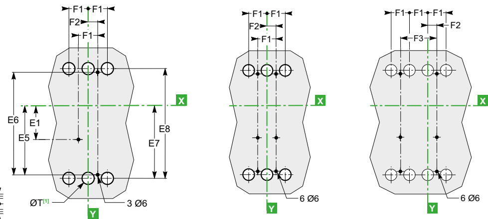
NSX100 à 250
