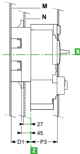
Avec bascule
