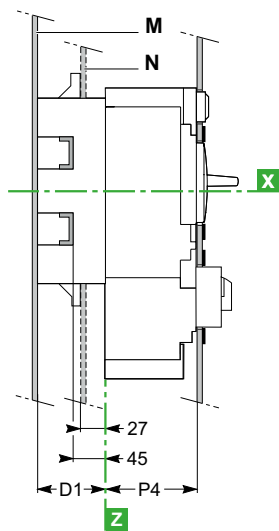
Commande par maneton
