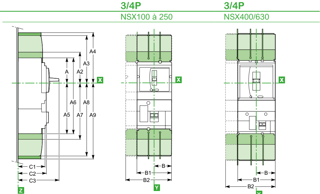
NSX100 à 250
