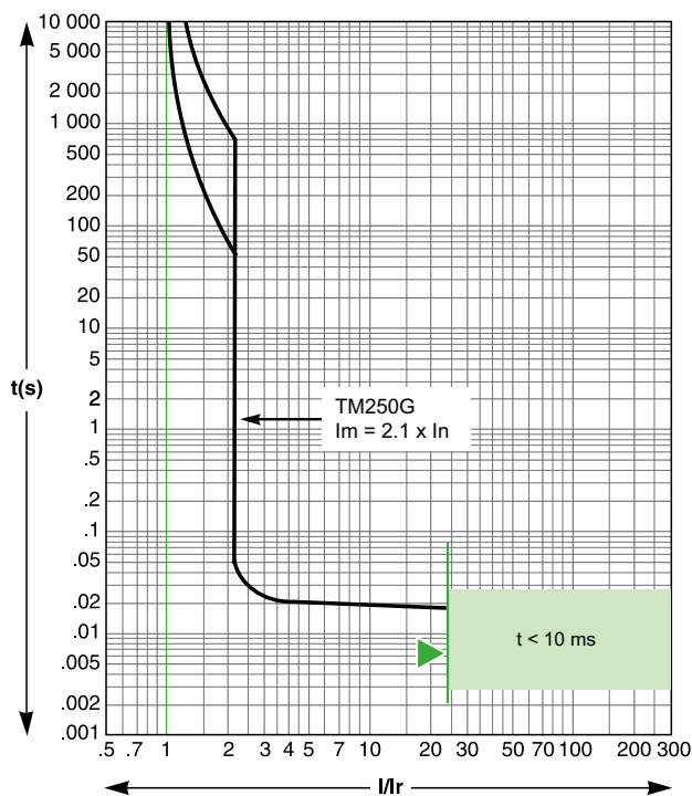
TM250G
