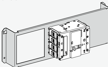
Montage sur une plaque de montage Prisma.
