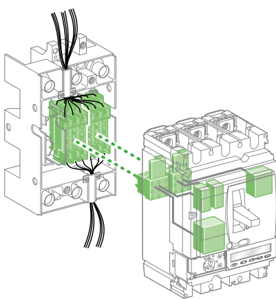
ComPact NSX débrochable.
