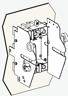
Fixation sur panneau arrière.
