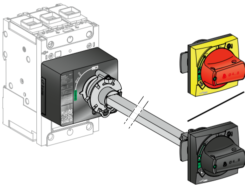
Commande rotative montée sur porte.
