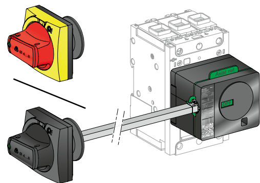
Commande rotative en montage latéral.
