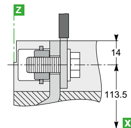
Barres/câbles avec cosses
