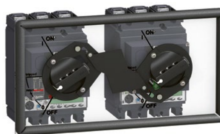
Verrouillage de deux appareils par commandes rotatives.
