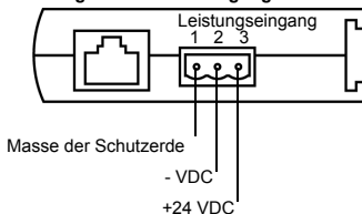
Stromanschluss
