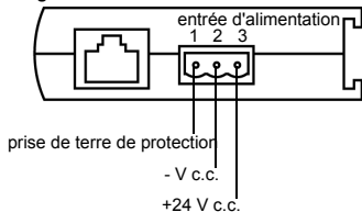
connecteur d'alimentation
