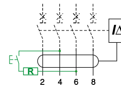
Example Vigi iC60
