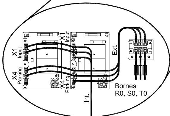
Cableado de salida de fábrica: ventiladores con alimentación interna por R/L1, S/L2, T/L3
