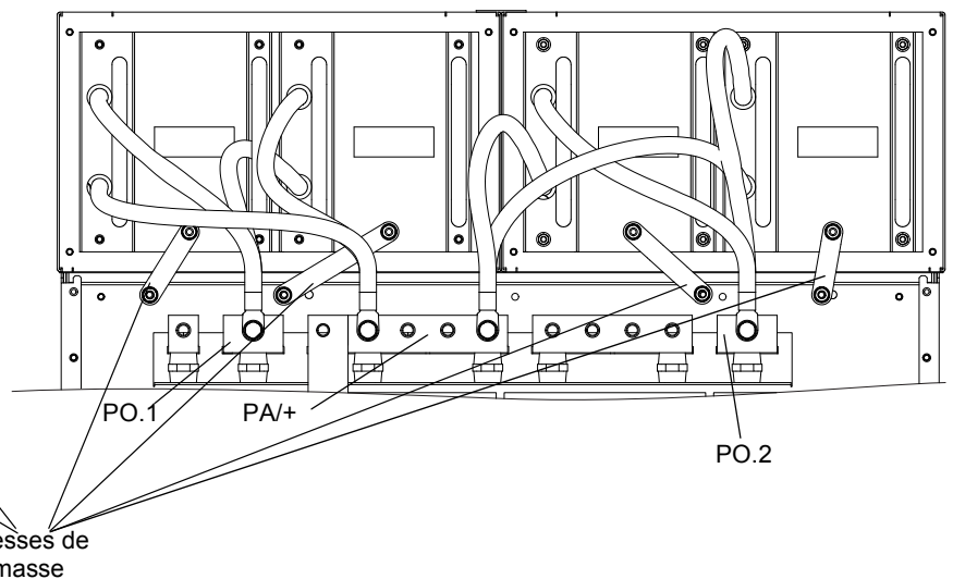
Exemple 4 : ATV61H C50N4 ... C63N4
