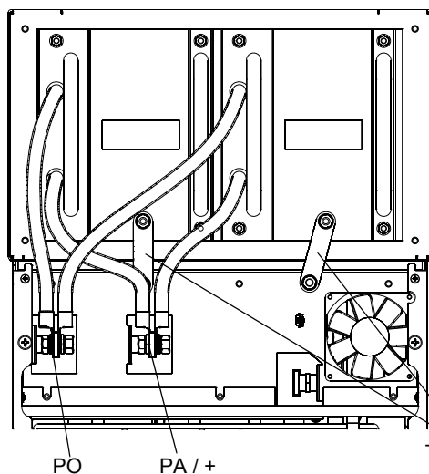
Exemple 2 : ATV61H C22N4 ... C31N4
