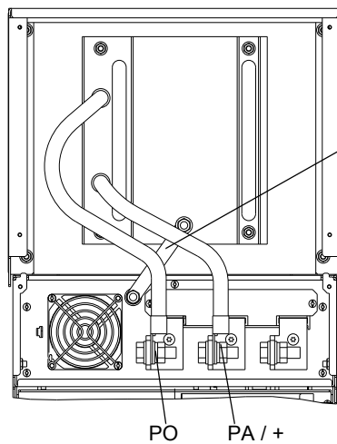
Exemple 1 : ATV61H D55M3X ... D90M3X, ATV61H D90N4 ... C16N4
