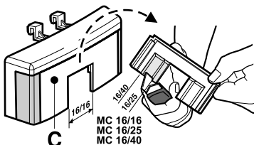
Opciones como adaptador lateral / Options as side adapter
