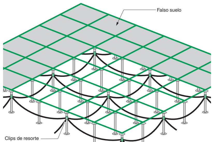
Fig. Ap8: Instalación de falso suelo.
