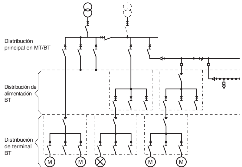
Fig. D2: Ejemplo de esquema unifilar.
