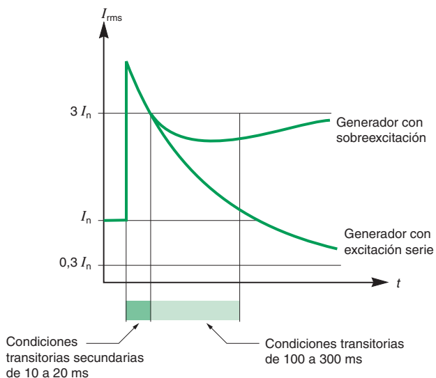
Fig. N27: Generador durante cortocircuito.
