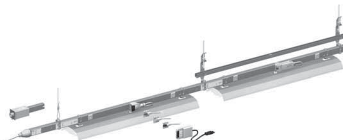
Fig. E61: Canalización eléctrica prefabricada rígida portadora de luminarias: Canalis KBA o KBB (25 y 40 A).
