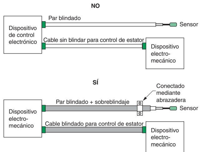
Fig. Ap32: Protección y sobreprotección de los cables sensibles y/o de perturbación.
