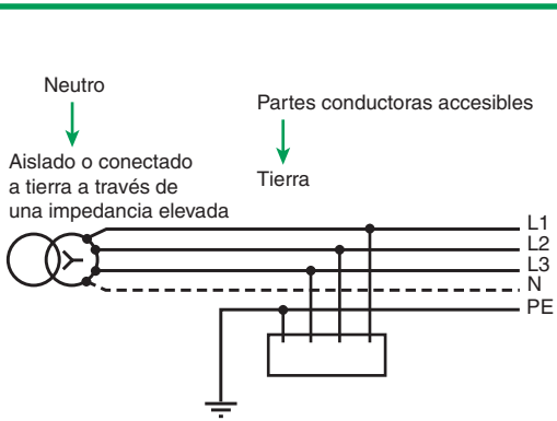
Fig. E29: Esquema IT (neutro aislado).
