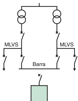
Fig. D22: Cuadros de distribución interconectados.
