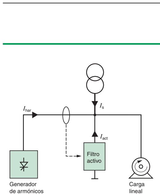
Fig. L28: Principio de funcionamiento del filtro activo.
