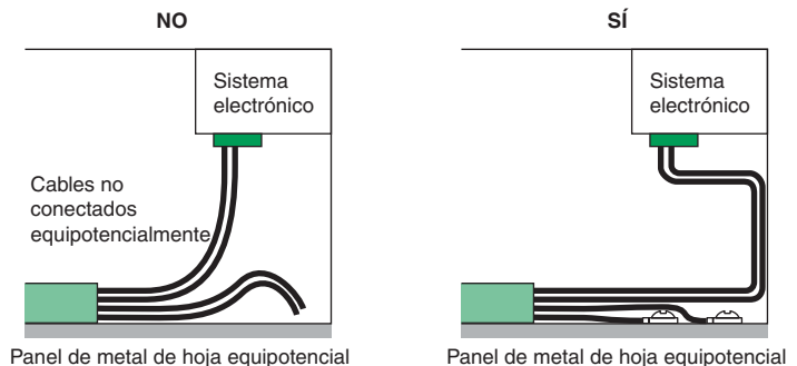
Fig. Ap34: Los cables libres deben estar conectados equipotencialmente.
