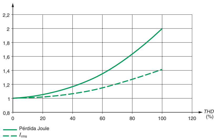
Fig. M8: Aumento en la corriente rms y en las pérdidas Joule como una función de THD4.
