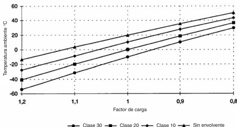
Fig. B33b: Curvas para transformadores con aislamiento seco.
