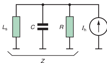
Fig. M7: Diagrama equivalente a la instalación que se muestra en la Figura M6 .
