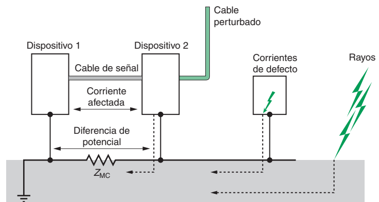
Fig. Ap20: Ejemplo de acoplamiento por impedancia en modo común.
