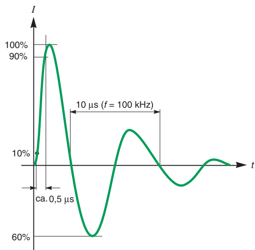
Fig. F68: Onda de corriente transitoria de 0,5 \mu s/100 \text{ kHz} normalizada.
