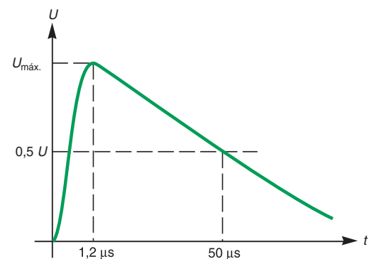
Fig. F69: Onda de tensión transitoria de 1,2/50 \mu s normalizada.
