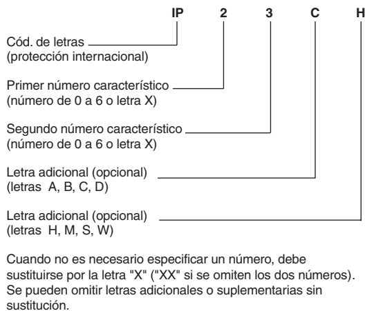
Fig. E66: Organización de los códigos IP.
