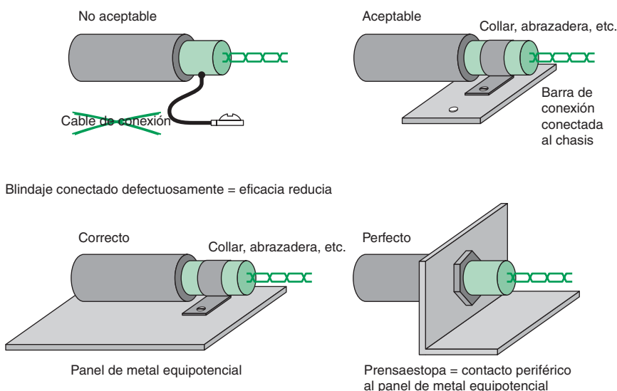
Fig. Ap15: Instalación de cables blindados.
