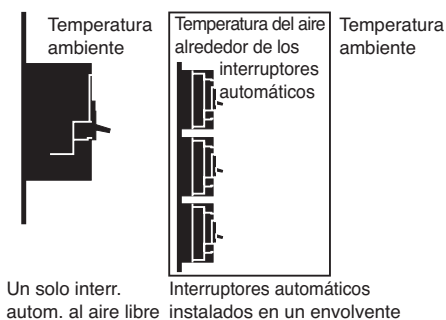
NS250N/H/L (temperatura de referencia: 40 °C)
