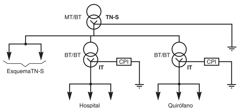
Fig. E40: Islas IT en un esquema TN-S.
