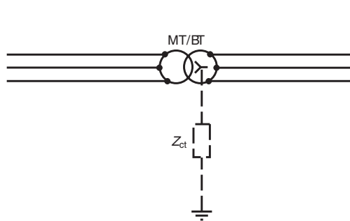
Fig. E31: Impedancia equivalente a las impedancias de fuga en un esquema IT.
