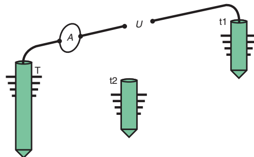
Fig. E46: Medición de la resistencia a tierra de la toma de tierra de una instalación mediante un amperímetro.
