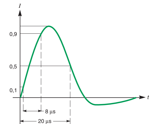
Fig. F70: Onda de impulso de corriente normalizada 8/20 \mu s .
