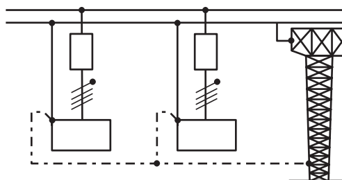
Fig. F54: Conexión equipotencial mejorada.
