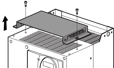
取下用于以下变频器的保护性冲裁盖板： ATV 21HD22M3X, HD30M3X, ATV 21HD22N4, HD75N4
