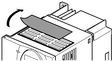
取下用于以下变频器的保护性冲裁盖板： ATV 21H075M3X...HD18M3X, ATV 21H075N4...HD18N4
