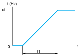
线性加速斜坡
