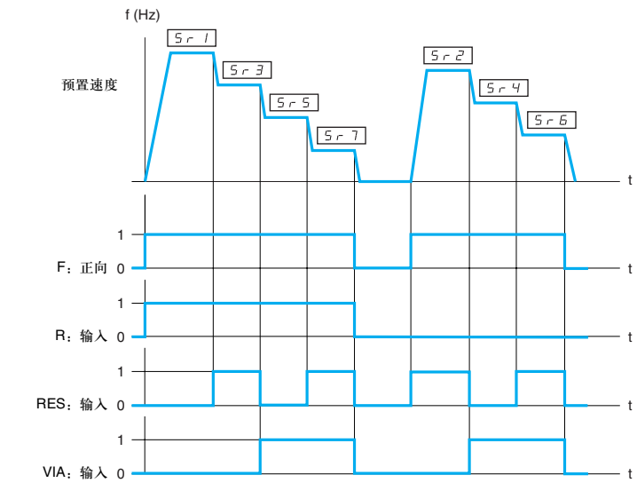
具有 7 种预置速度的运行示例
