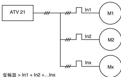
变频器 > In1 + In2 + ... Inx 电机并联
