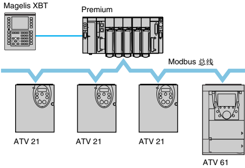
Modbus 总线配置示例
