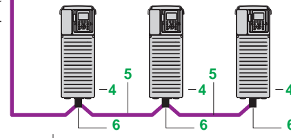
Преобразователь частоты Altivar Process + модуль связи WW3A3618
