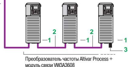
Шина CANopen (3)
