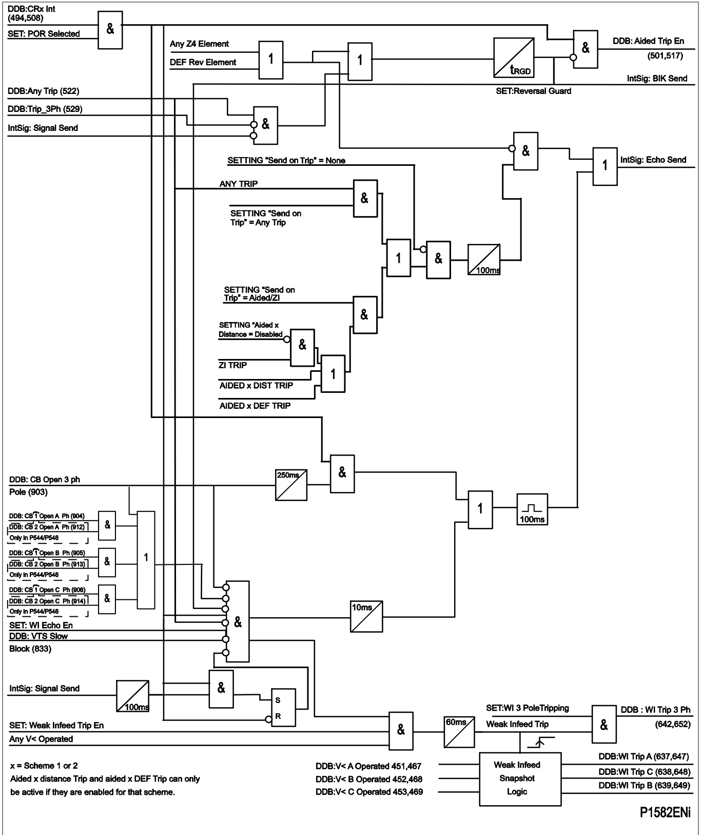
Figure 43 - POR Permissive OverReach
