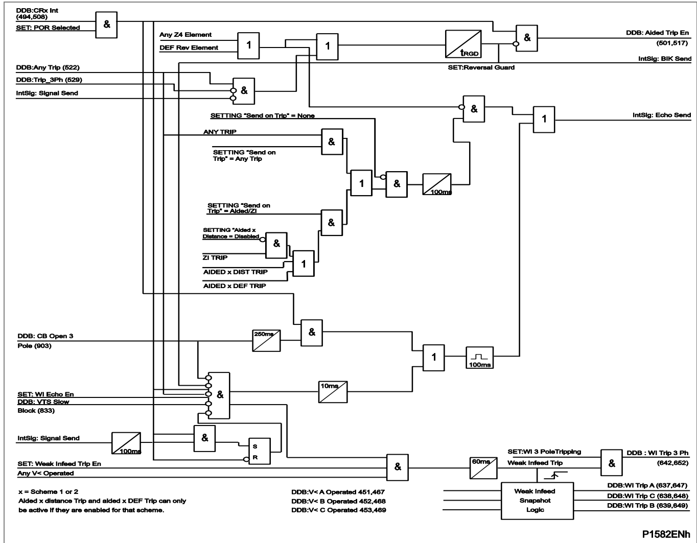
Figure 25 - POR
