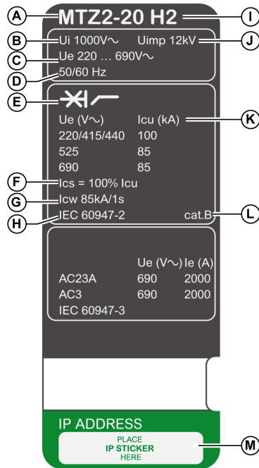
Placa de características del interruptor automático
