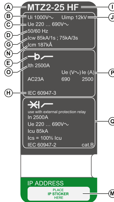
Placa de características del interruptor en carga
