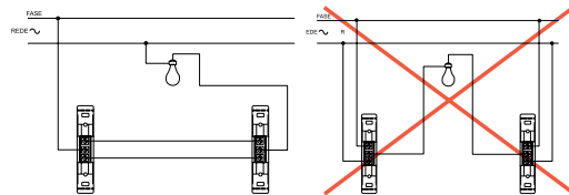
Ligação de interruptor paralelo correta
