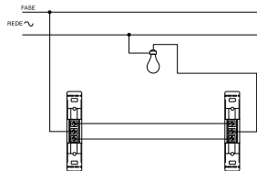
Ligação de interruptor paralelo correta
