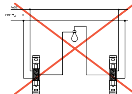
Ligação de interruptor paralelo não recomendável
