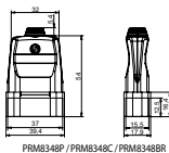
Tomada móvel 2P cilíndricos 10A 250V--
